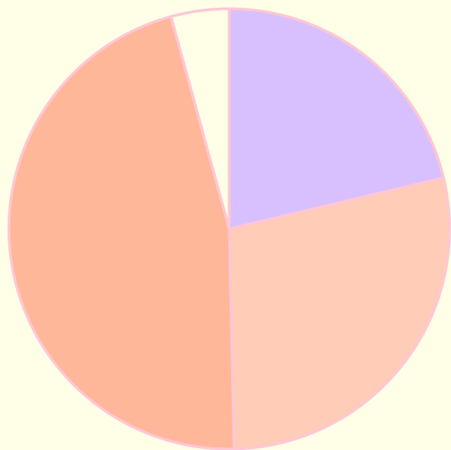
Распределение баллов
